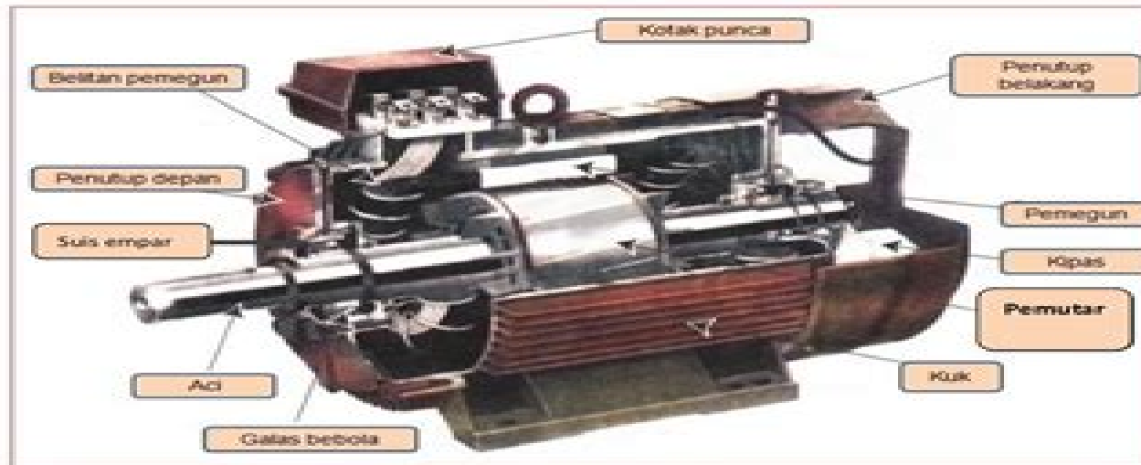
Bahagian dalam Motor aruhan 3 fasa sangkar tupai
