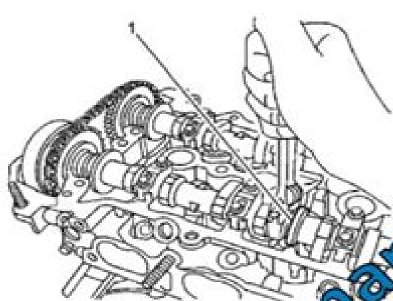
Fig. 109: Holding Camshaft
