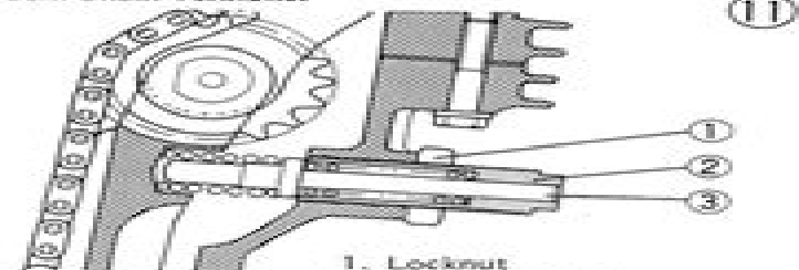
1. Locknut 2. Push Rod Guide 3. Push Rod
