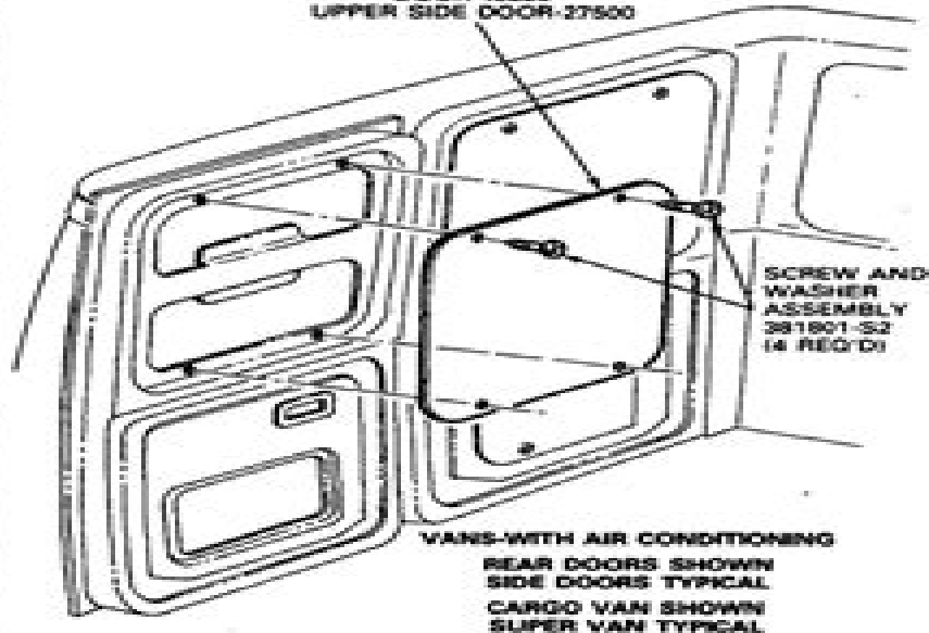
FIG. 9 Cargo Van Hinged Door Panel—Rear
