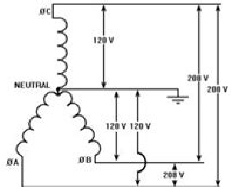
208Y/120 V
