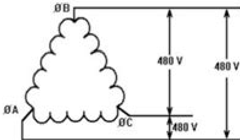
480 V Delta
