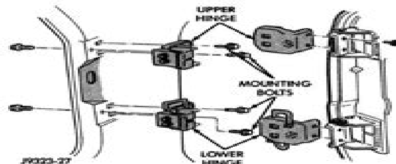
Fig. 15 Door Hinges and Bolts
