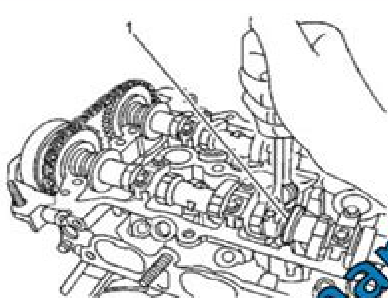
Fig. 109: Holding Camshaft
