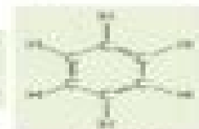
Benzene
