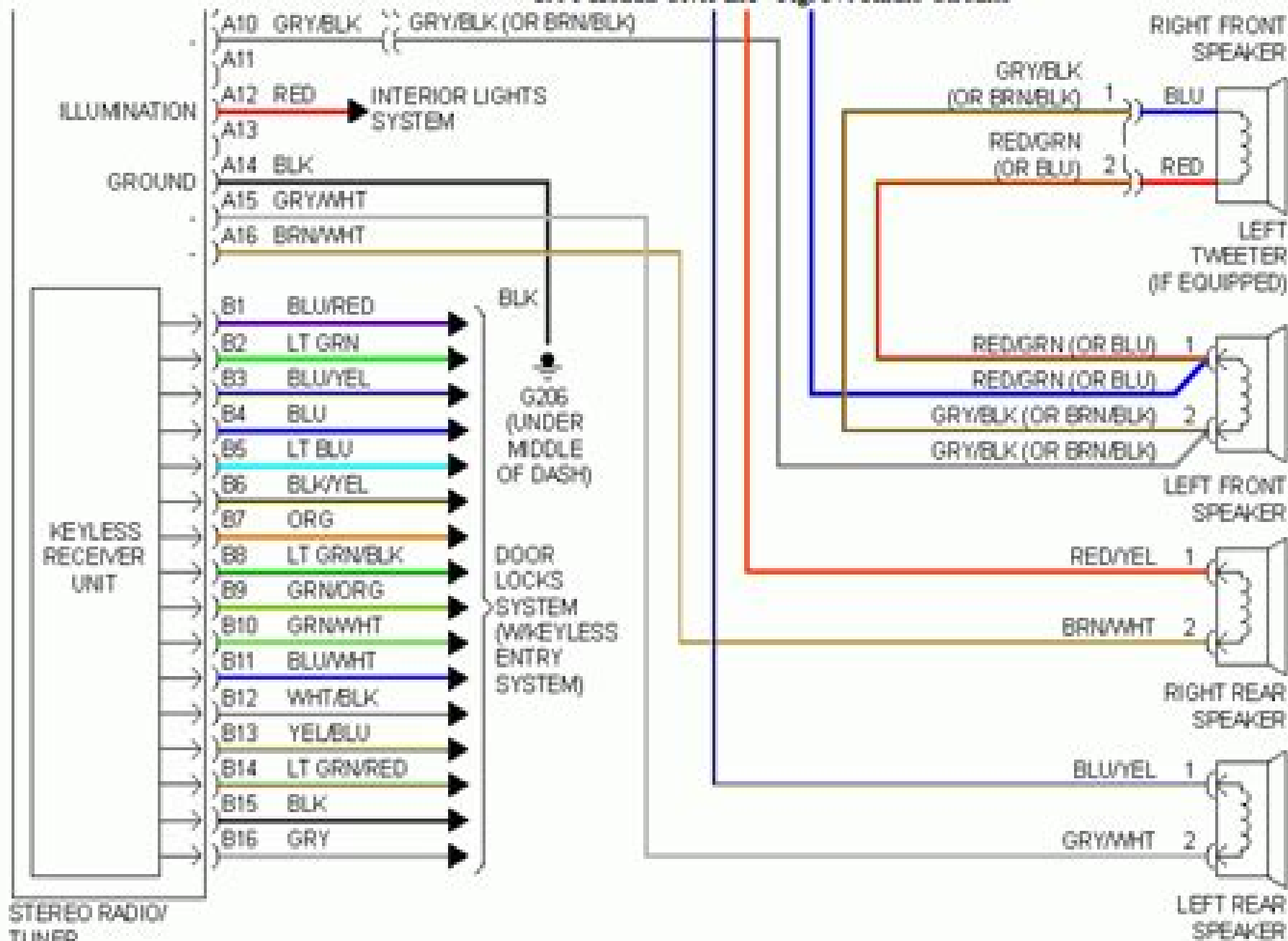
1996 Honda Civic LX - Fig. 37: Radio Circuits
