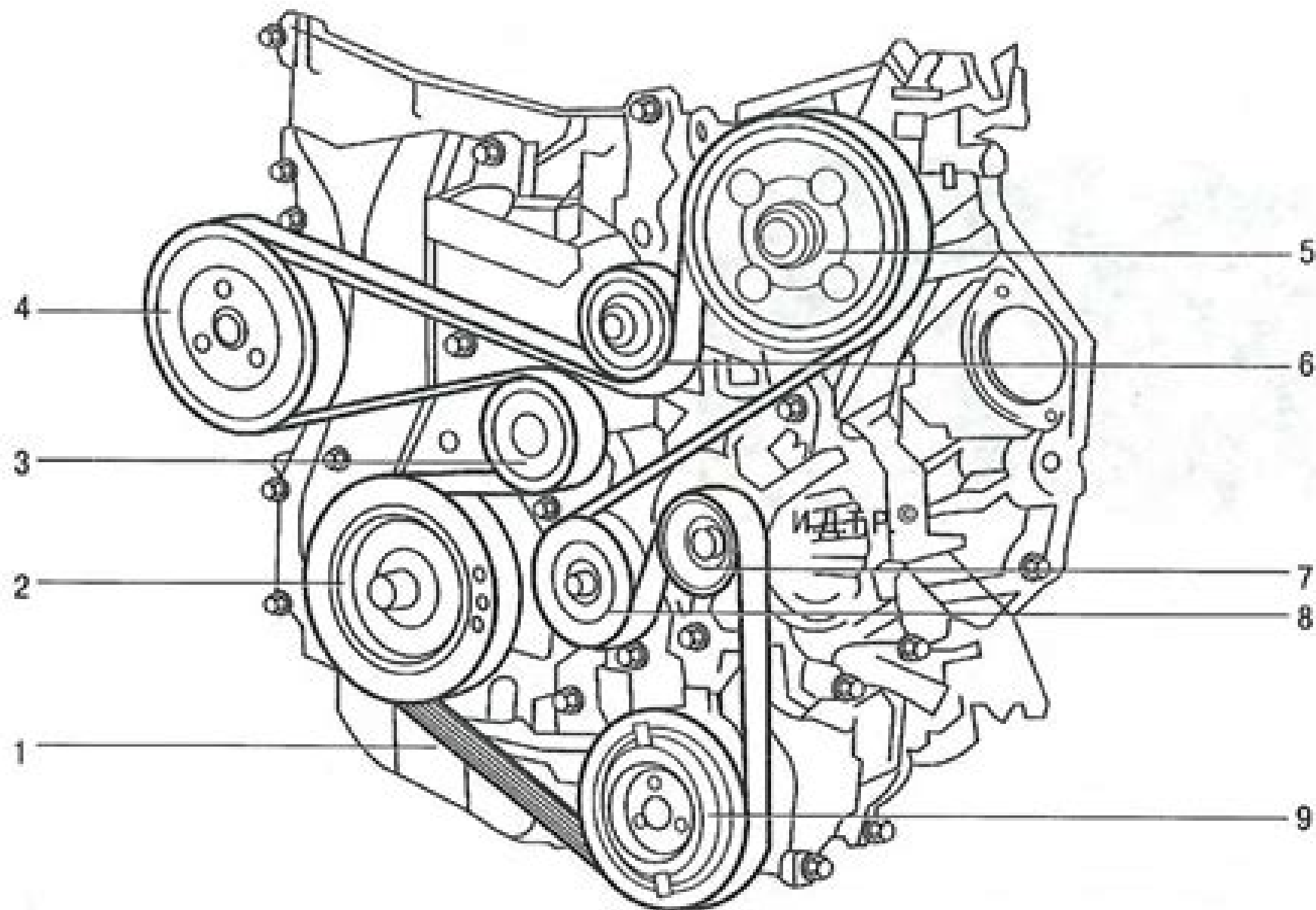
Рис. 5.29. Прокладка ремня привода вспомогательных агрегатов двигателя G4KD: 1 – ремень привода вспомогательных агрегатов; 2 – шкив коленчатого вала; 3 – натяжное устройство; 4 – шкив водяного насоса; 5 – шкив насоса гидроусилителя рулевого управления; 6, 8 – направляющие ролики; 7 – шкив генератора; 9 – шкив компрессора кондиционера
