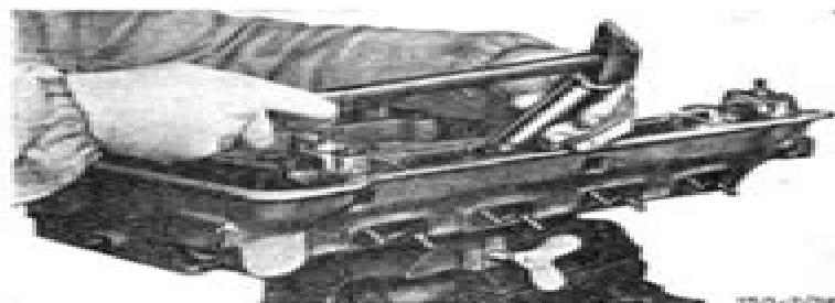
Abb. 56. Einbau der Ventilführungsbüchsen mittels Werkzeug 6121.07.291.
