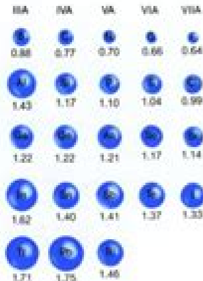
Ionic Radii
