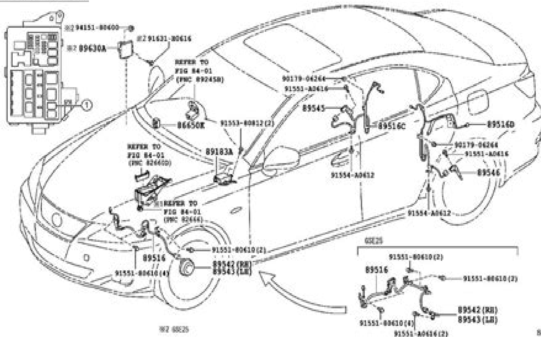
図1 エンジンルーム リレーボックス
