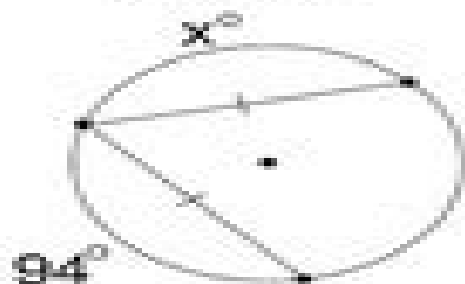
Arcs
