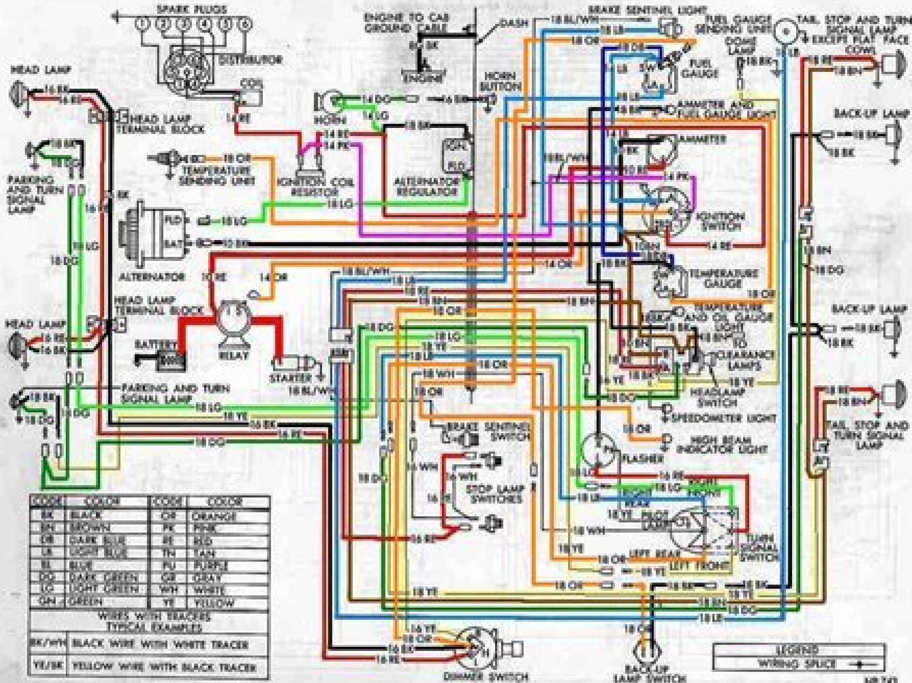
WM300 Body Wiring
