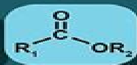
ESTER
