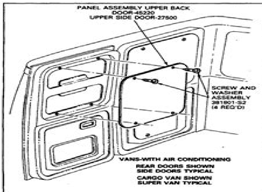
FIG. 9 Cargo Van Hinged Door Panel—Rear
