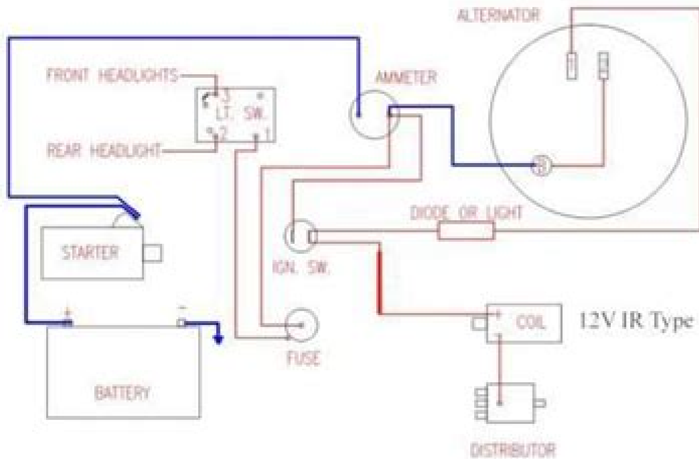
12 VOLT DIAGRAM
