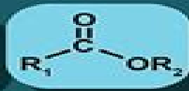
ESTER
