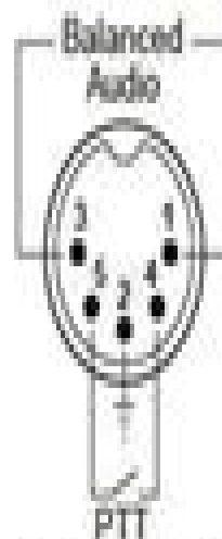
C 0376 5 Pin DIN Wiring Diagram
