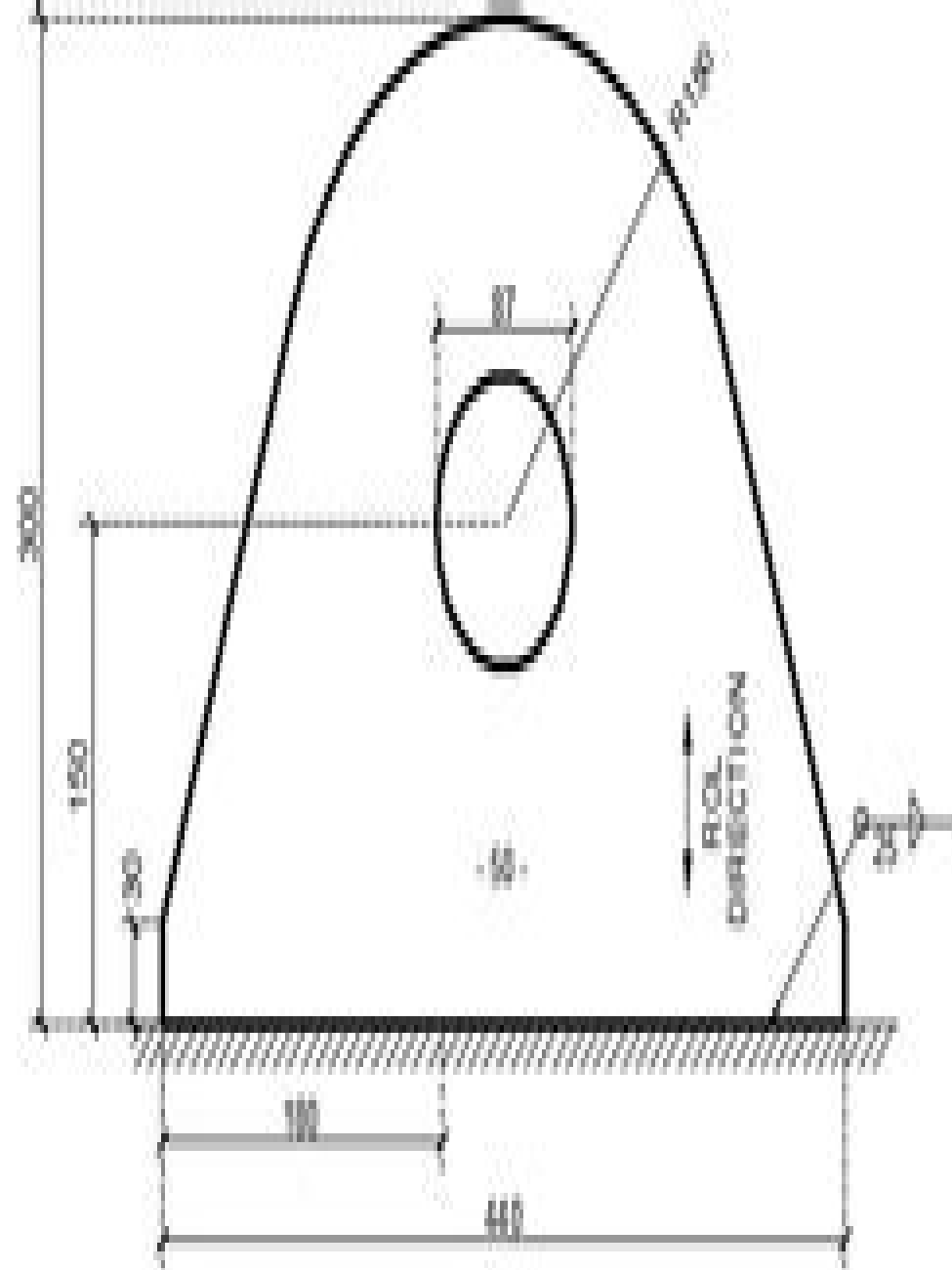
PADEYE - 85 mT
