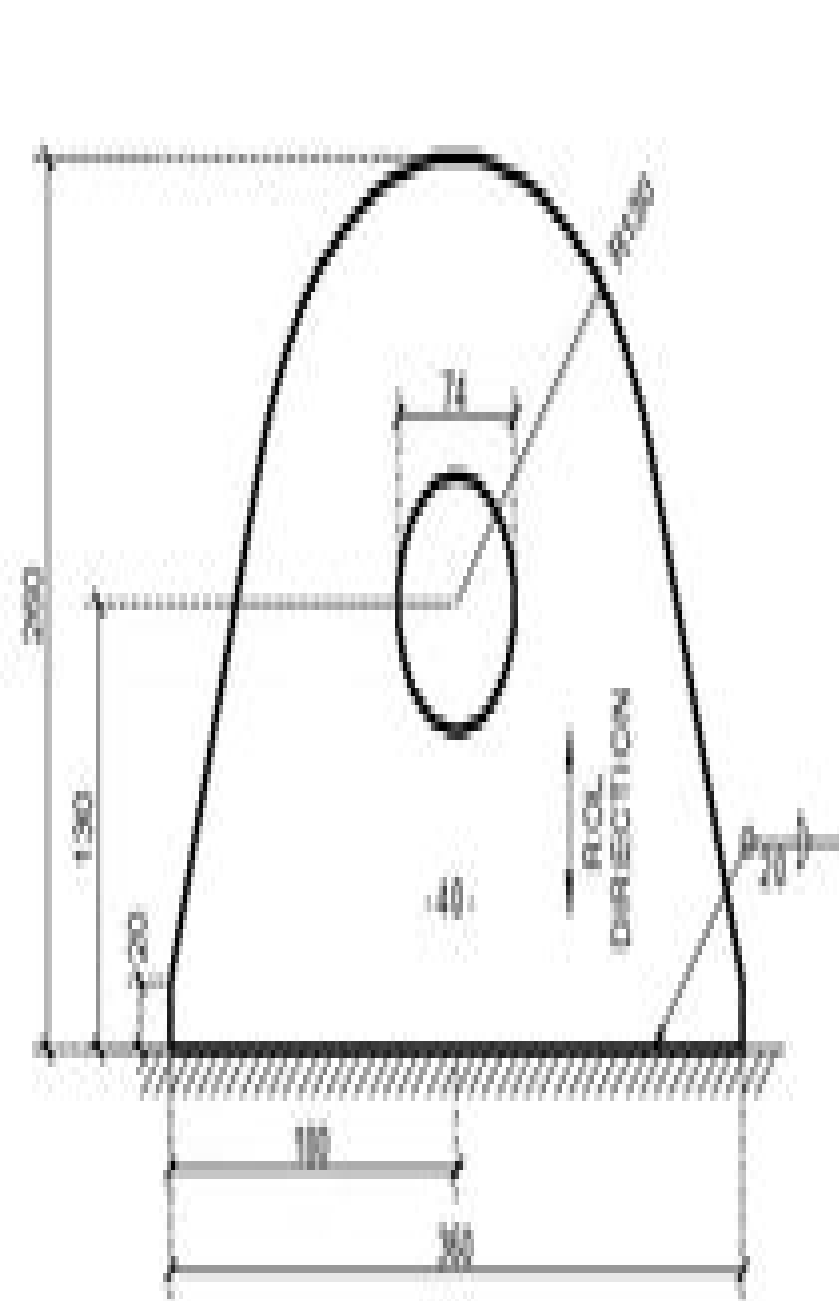
PADEYE - 55 mT
